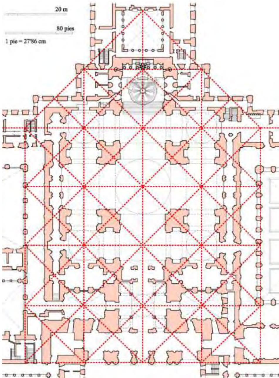
Comprobación del trazado de la Basílica modulada según sus ejes; la modulación se extiende a las fachadas del patio de mascarones, el retablo, la Basílica y los claustros (dibujo del autor).
