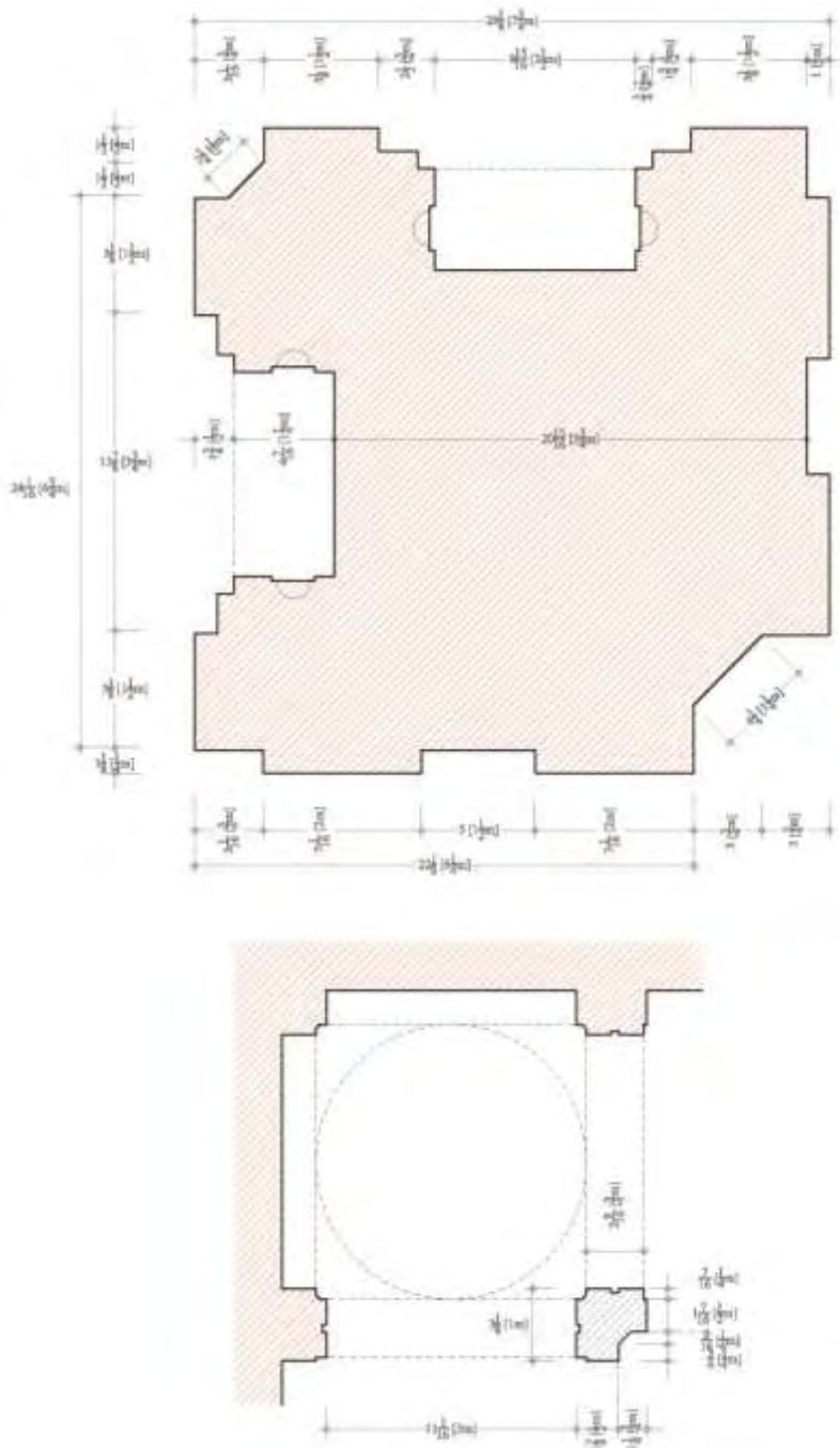
Mediciones en pies y en metros de los pilares centrales de la Basílica de El Escorial, tomando un pie de 27,86 cm, comparados con los de la bóveda plana. Las cotas se dan a un metro de la cota del solado (mediciones y dibujo del autor).
