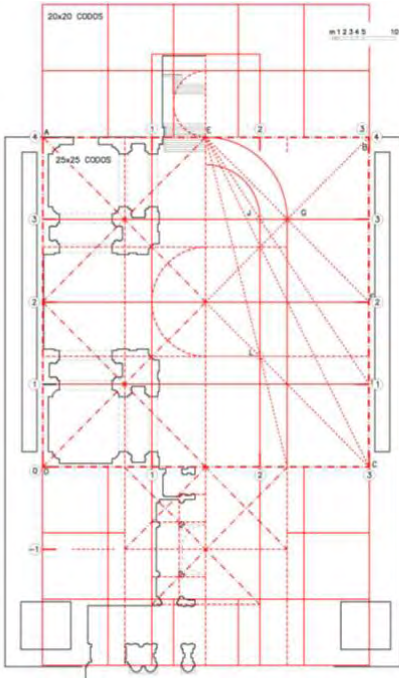
Hipótesis del trazado de la Basílica, superponiendo las tramas de 5x5 (la original de 20x20 codos) y la doble de 4x4 y 3x3. El trazado no se habría hecho por adición de módulos (método clasicista) sino por ejes, según la tradición medieval de Rodrigo Gil (dibujo del autor).
