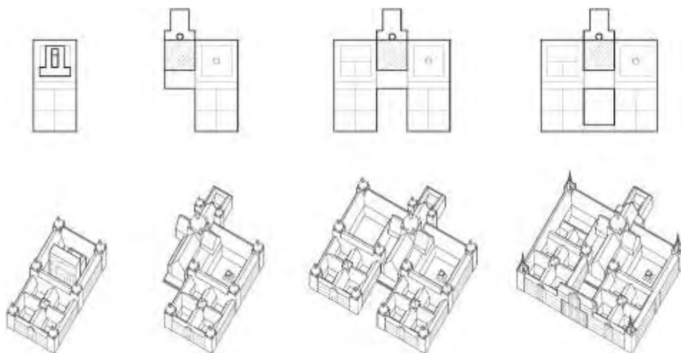
1. Hipótesis básica «salomónica» 2. El Monasterio reducido al esquema monacal tradicional (según F. Chueca). 3. El Monasterio completado, sin cerrar el atrio del templo, según las trazas conservadas del proyecto original. 4. Solución definitiva de Juan de Herrera, con chapiteles, la biblioteca en la entrada y simplificando las torres (dibujos del autor)
