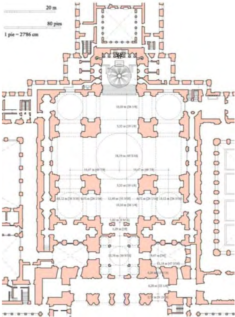
Mediciones en pies y en metros de la Basílica, con un pie de 27,86 cm, con la separación entre naves, bóveda plana y patinejos. Las cotas están tomadas a un metro de la cota del solado (mediciones y dibujo del autor).
