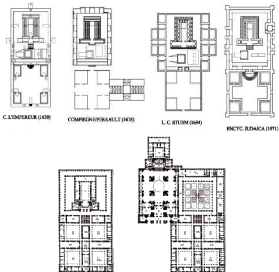
Cuatro reconstrucciones del Templo de Jerusalén, siguiendo la descripción de Josefo. Comparación con mi hipótesis salomónica y con la hipótesis morfogenética de F. Chueca.
