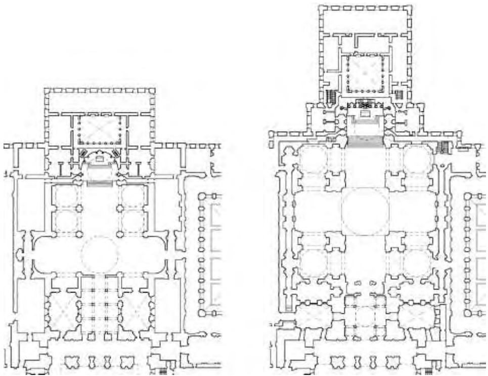
Hipótesis de la planta original junto a la versión definitiva de la Basílica. Dibujo del autor
