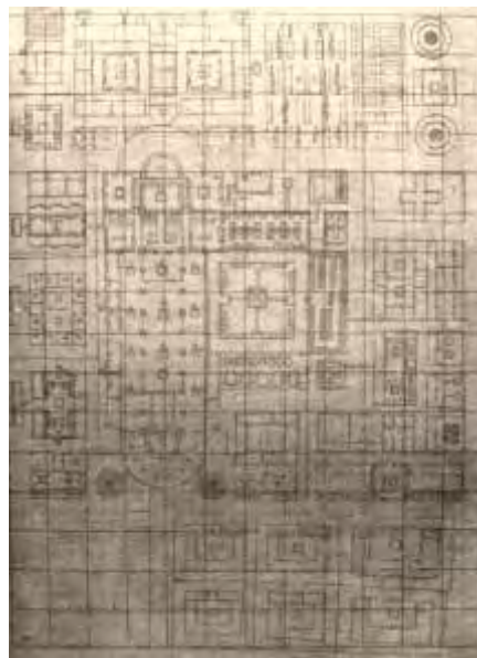
Esquema básico del convento escorialense medido en codos. Plano de la abadía de San Galo, otro convento organizado sobre una cuadrícula de 40 pies de lado, según Horn y Born
